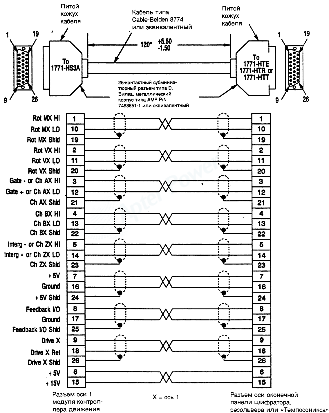
Рисунок А.1 Спецификации кабеля 1771-CAE и схема подключения
